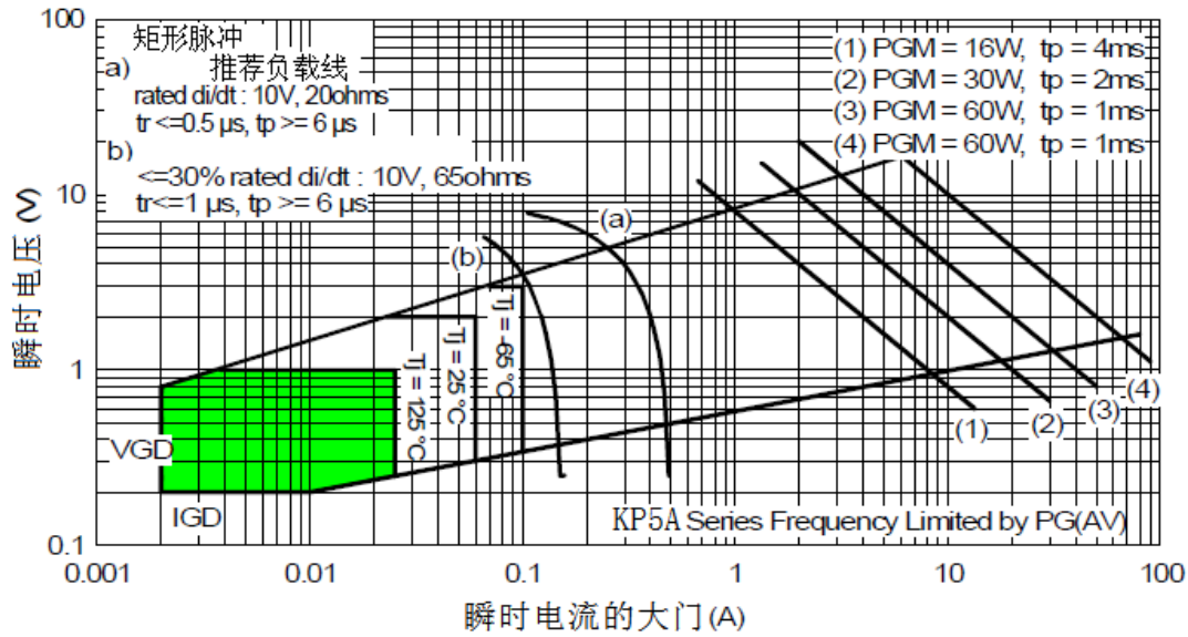
Fig. 16 - 栅极特性
