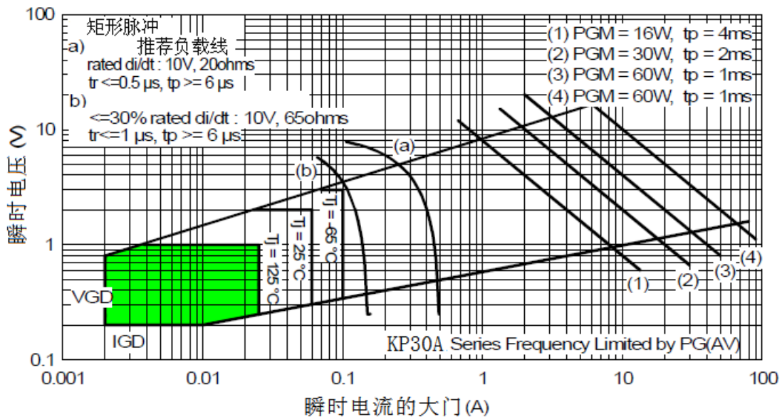
Fig. 16 - 栅极特性
