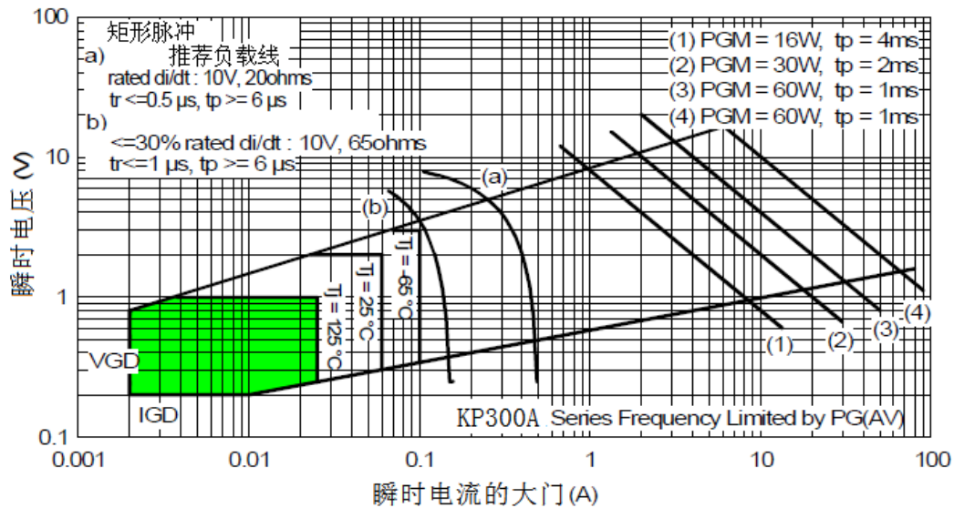
Fig. 16 - 栅极特性
